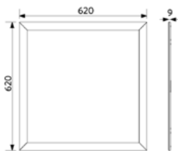
LEDPanelRc-S5 Re295
