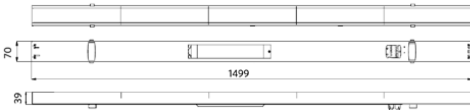
Tragschiene 8 Verbindungsstück
