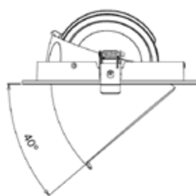
LEDSpotRS-P 35W
